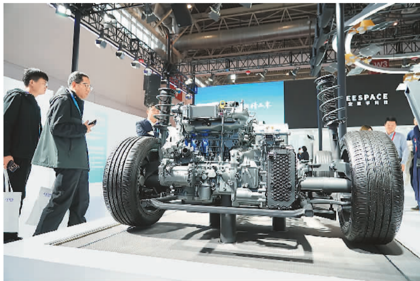
11月28日，在首届链博会智能汽车链展区，观众正在参观吉利汽车集团展位的“雷神”电混系统。
