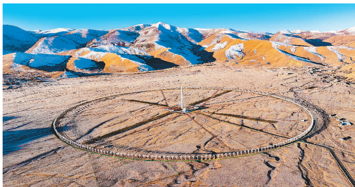
日前,四川省稻城县,雪山映衬下的圆环阵太阳射电成像望远镜壮丽如画。该望远镜今年通过工艺测试,是国家重大科技基础设施“空间环境地基综合监测网(子午工程二期)”的标志性设备之一,可为太阳物理和空间天气研究提供高质量观测数据。
