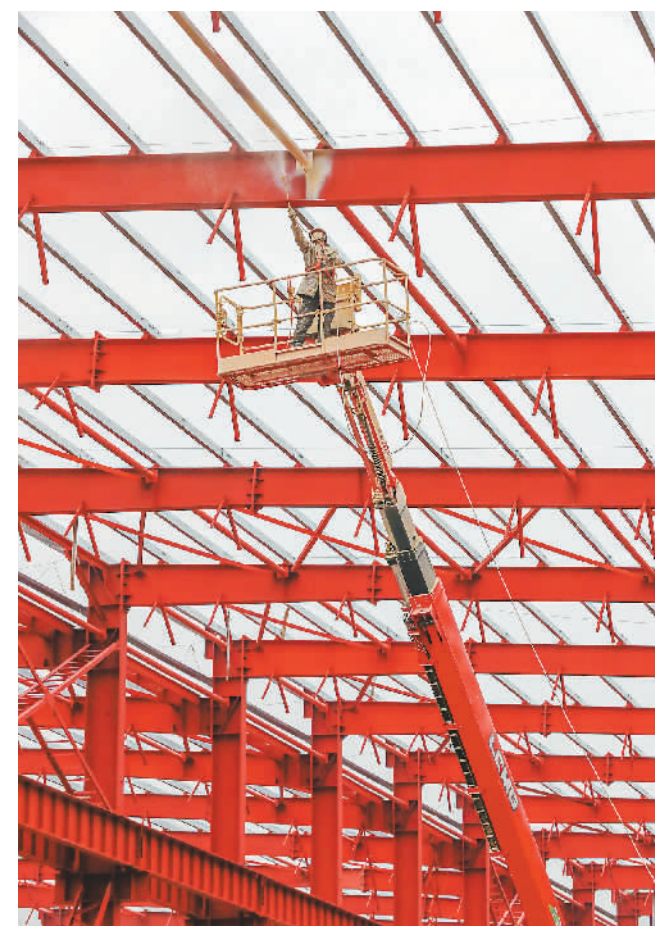
2月1日,在浙江省湖州市英干山高新区一高端轴承制造项目建设现场,工人们正在进行钢结构标准厂房施工。该项目主要承接新能源汽车轴承、大型工程机械重载轴承等产品,建成后 will 有力推动当地绿色智能制造产业集群发展。王树成摄(人民视觉)
