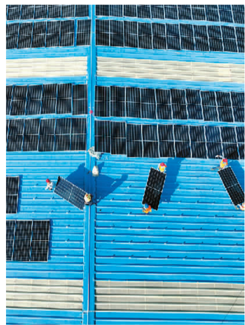
6月30日，湖北省十堰市房县北城工业园区厂房屋顶，施工人员在安装太阳能电池板。
