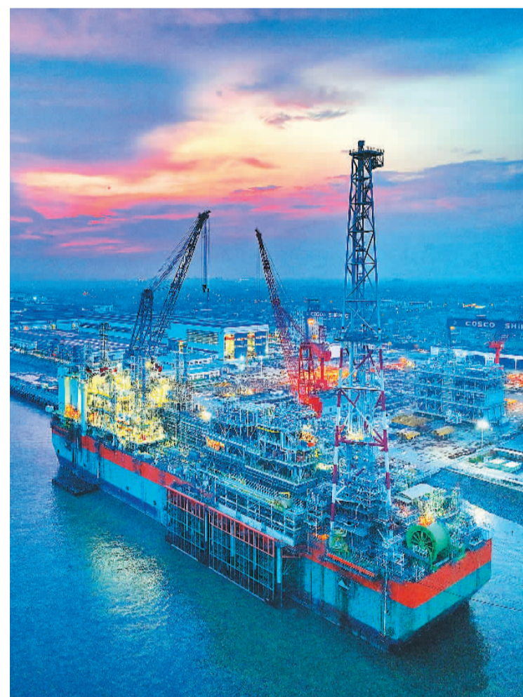
由江苏启东中远海运海工承建的浮式生产储卸油船N999项目目前调试接近尾声,下月将进行命名、试航。
