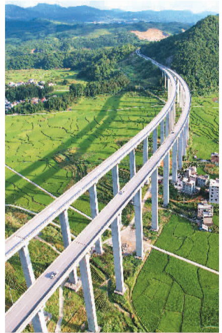
贵州省黔东南苗族侗族自治州从江县洛香镇黎从高速公路高架桥。石宏伟摄（人民视觉）
