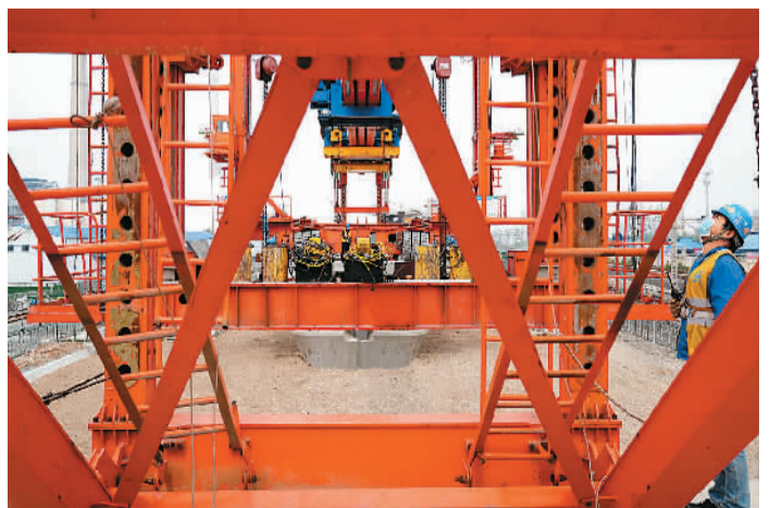
4月30日，山东省济南市黄台联络线施工现场，中铁十局的工作人员正在进行双线路架梁架桥作业。 新华社记者 郭 绪 雷 摄
