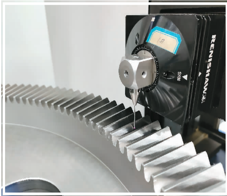
周元生团队在本次比赛中展示的面齿轮，高效精密智能制造中的在机测量关键技术。
