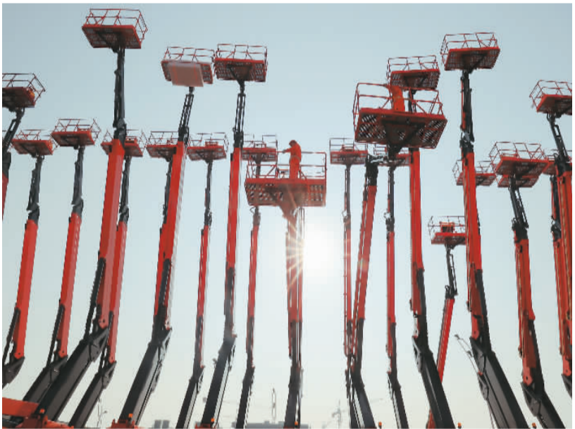
▲在位于浙江省湖州市德清县雷甸镇的一家机械制造企业，工人赶制今年出口海外的新臂式智能高空作业平台设备。 谢尚国摄（人民视觉）
