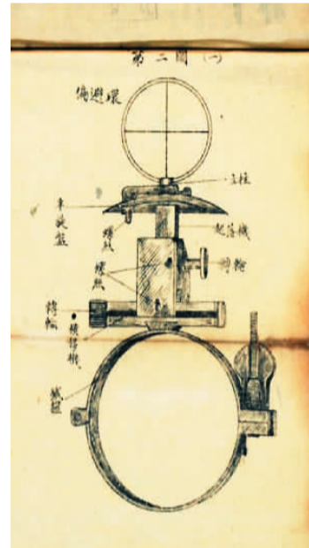
王智涛设计的高射机枪瞄准镜
