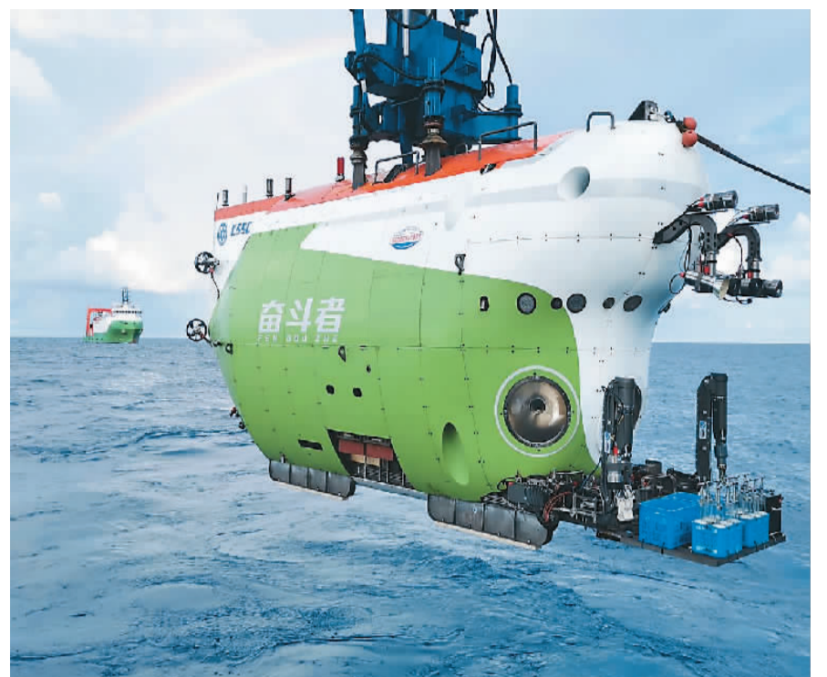
2020年11月28日,由中国船舶集团制造的创造了10909米中国载人深潜新纪录的“奋斗者”号,完成第二阶段海试,胜利返航。图为“奋斗者”号。中国船舶集团供图(新华社发)
