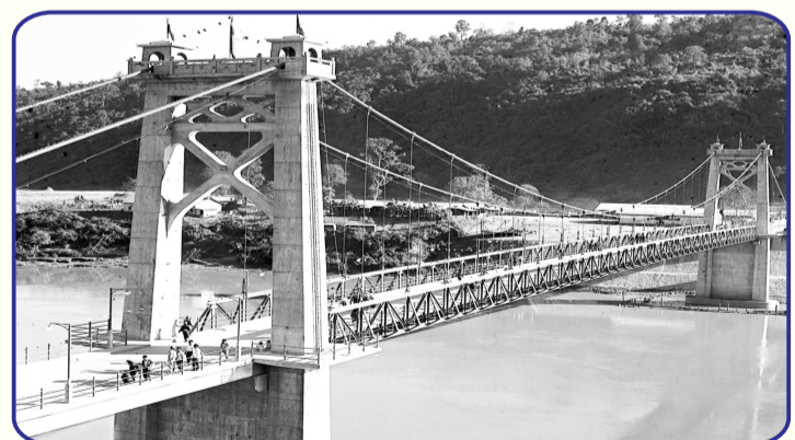
中国援建缅甸的滚弄钢索吊桥1965年建成通行,成为象征中缅两国人民之间友好合作的“友谊桥”。桥长247.9米,宽6.75米,桥上有一条汽车道,两条人行道,可容纳24辆满载10吨的卡车同时在桥上通行。
