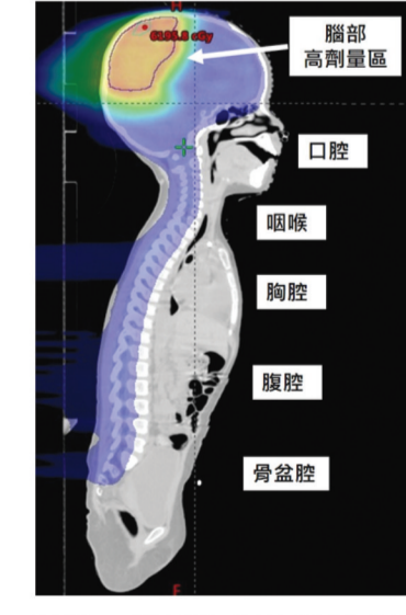
图说：质子治疗的剂量分布图，紫色区域是质子射束全脑全脊髓照射区域，可以看到从口腔、咽喉、胸腔、腹腔到骨盆腔，几乎没有治疗剂量的暴露；高剂量区为橘黄色区域，可以很明确的局限在手术区而不增加其它脑部的暴露剂量。
