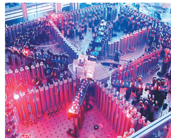
12月4日,中国科学技术大学宣布该校潘建伟等人成功构建76个光子的量子计算原型机“九章”,图为光子干涉实验图。
