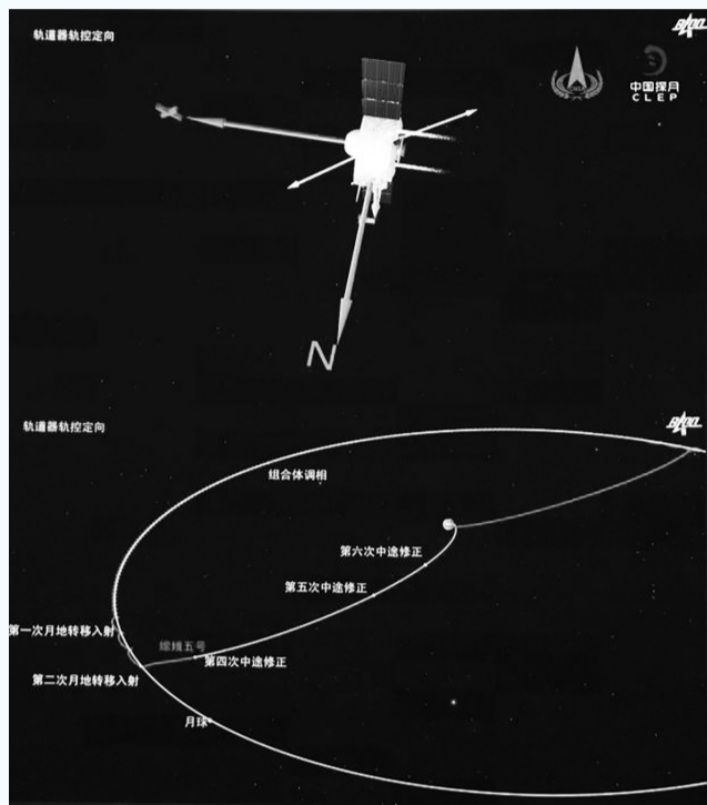
12月14日,嫦娥五号探测器轨控示意图。图片提供:国家航天局
